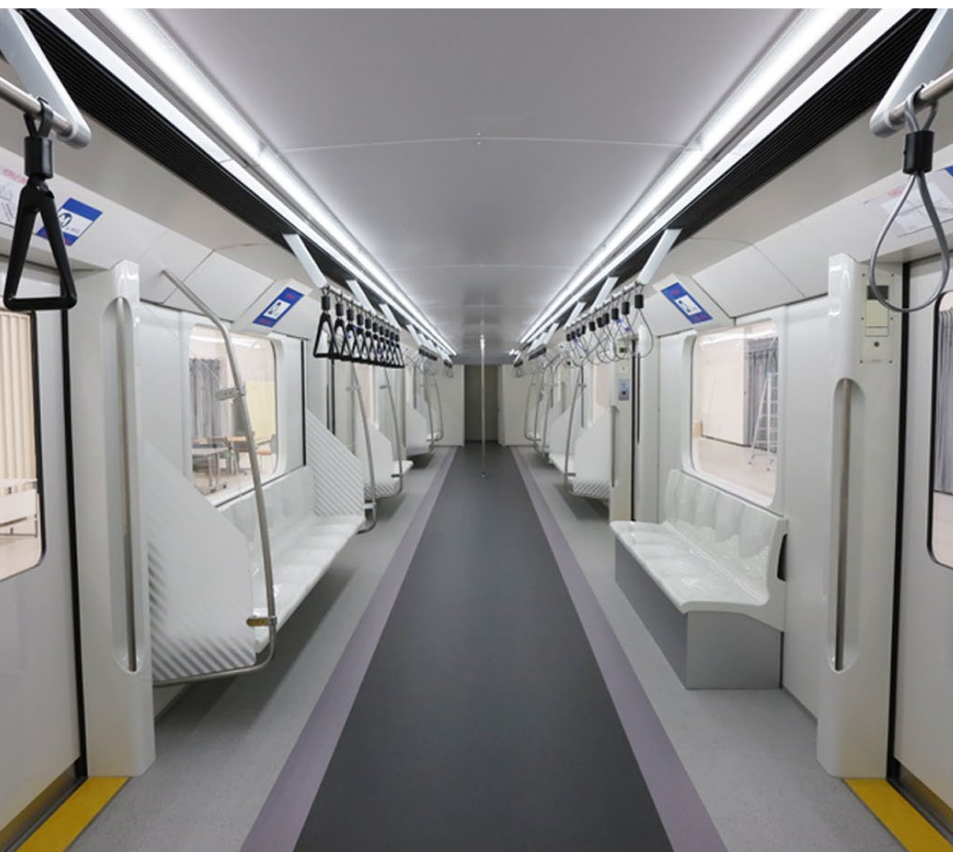
寸法：全長(AL)21.7m×全幅(AW)3.15m×全高(AH)2.74m
